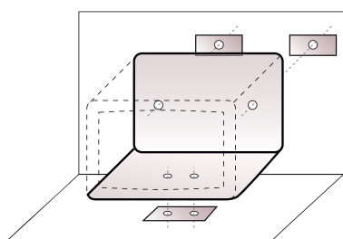
FISSAGGIO: 2 FORI SUL FONDO + 2 FORI SUL RETRO (TASSELLI DI FISSAGGIO INCLUSI). FIXING: 2 HOLES ON THE BOTTOM + 2 HOLES ON THE BACK (FIXING DOWELS INCLUDED).
