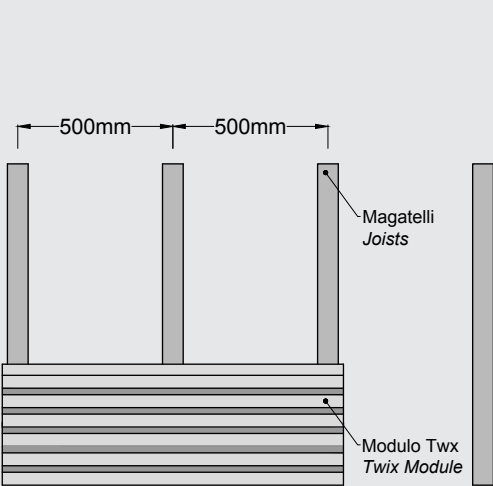
Installazione orizzontale / Horizontal installation
