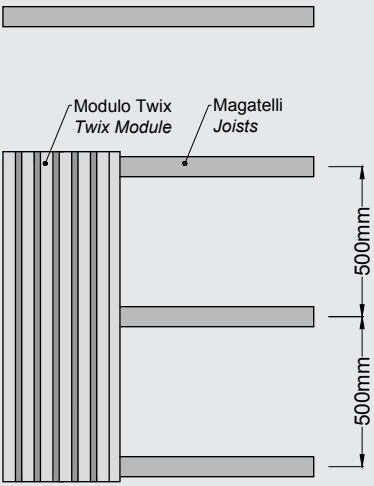
Installazione verticale / Vertical installation
